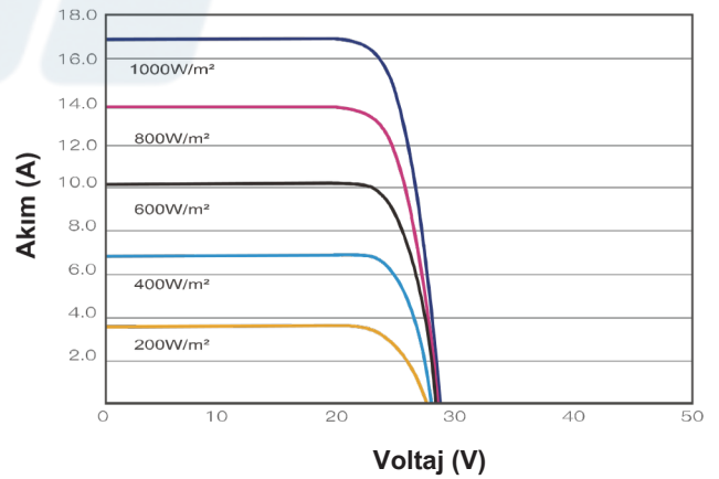
Akım - Voltaj Grafiği ( CWT395-80PM12-F )
